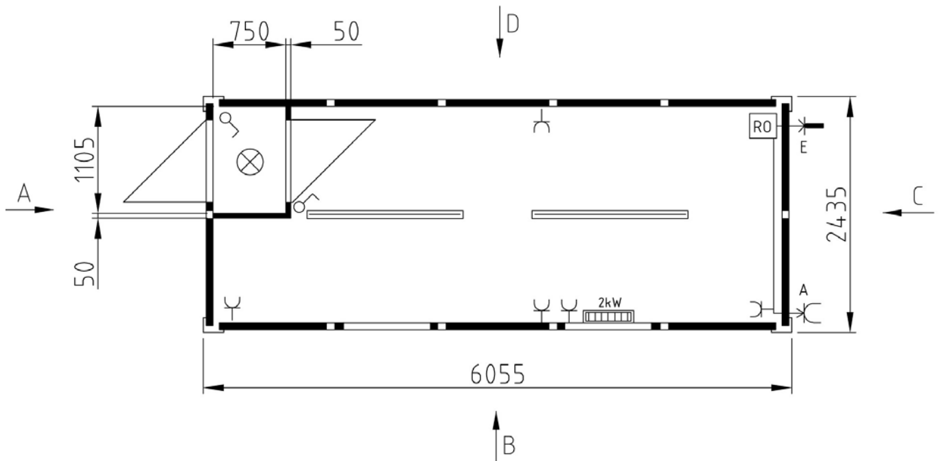
Ansicht A
